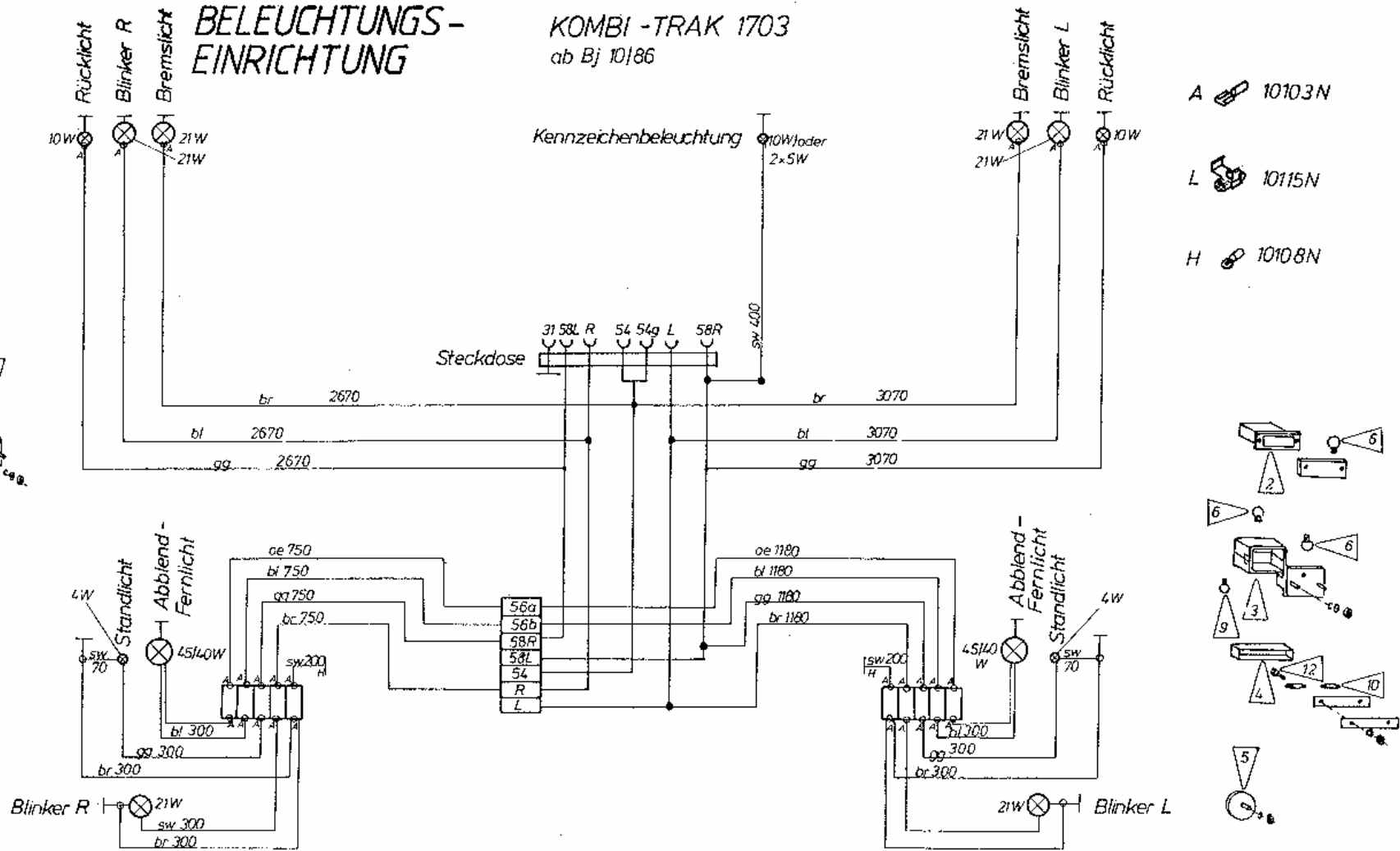
Kabellängen für Kombi Trak 170.3
